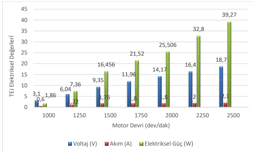
Şekil 7. TEJ sistemi tarafından üretilen elektriksel büyüklükler
