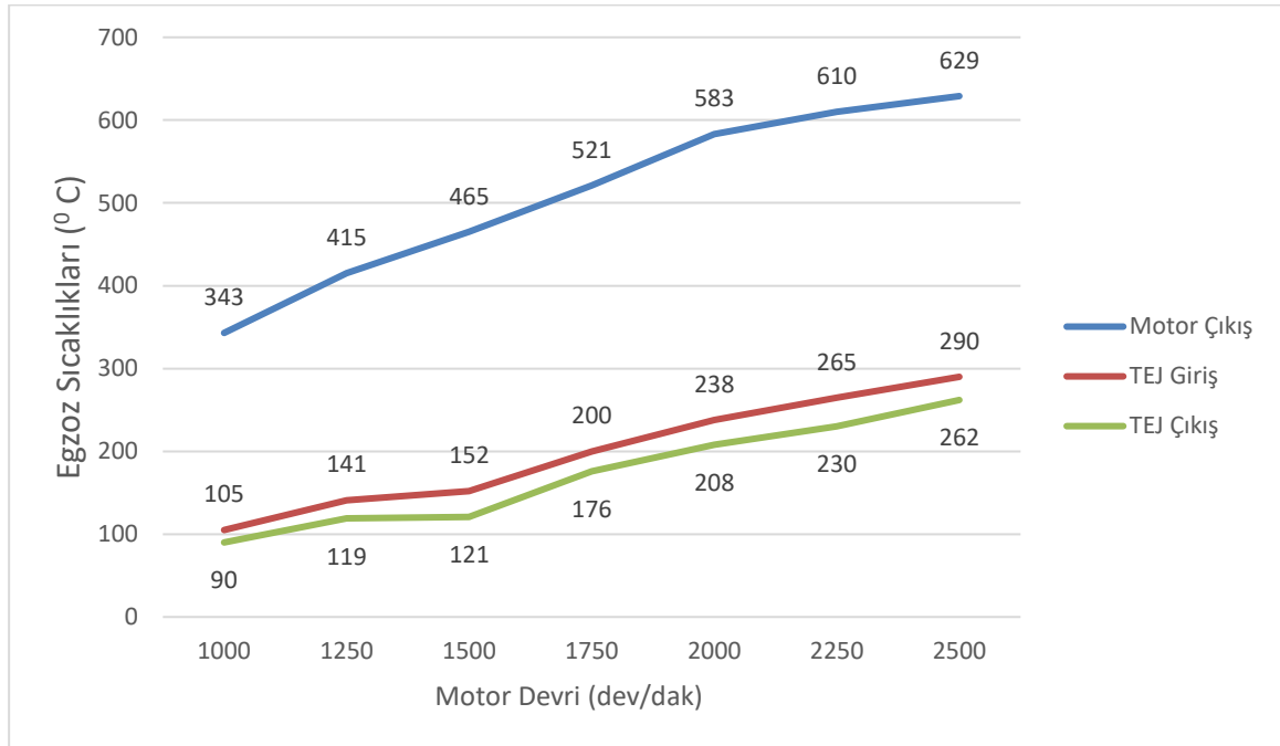
Şekil 5. Ölçülen egzoz sıcaklık değerleri
