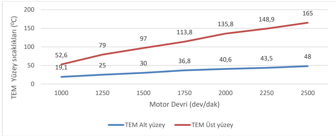
Şekil 6. TEM alt ve üst yüzey sıcaklıkları
