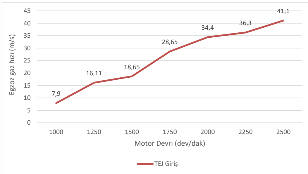
Şekil 4. Motorun farklı devirlerinde ölçülen egzoz gaz hızları
