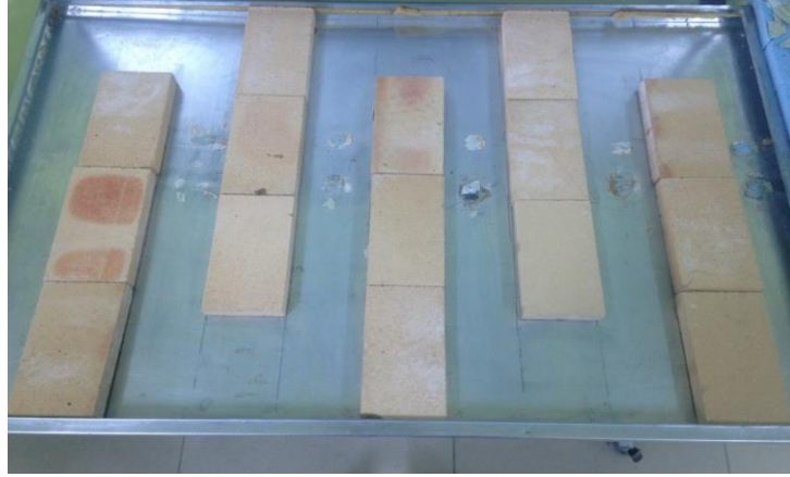
Şekil 5. Dolomit tuğlası kullanılan kollektör tasarımı
