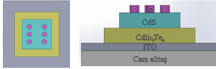
Şekil 1. Güneş Pili Şematik Yapısı
