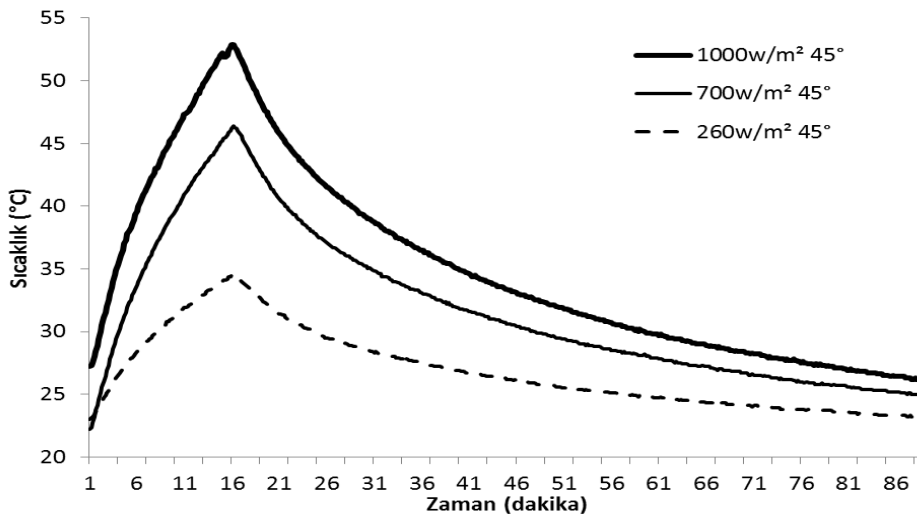
Şekil 6. 45^\circ geliş açısında kollektörden ölçülen sıcaklık değerlerinin değişimleri
