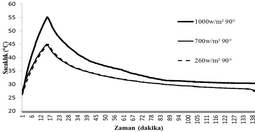
Şekil 7. 90° geliş açısında kollektörden ölçülen sıcaklık değerlerinin değişimleri
